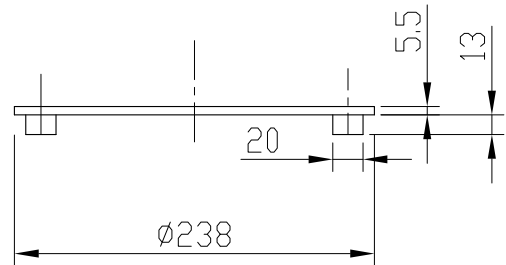
グレーチング
